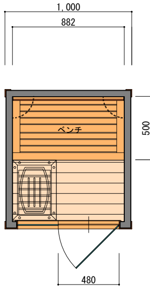
平面図 S=1/30
