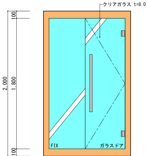
C 立面図 S=1/30
