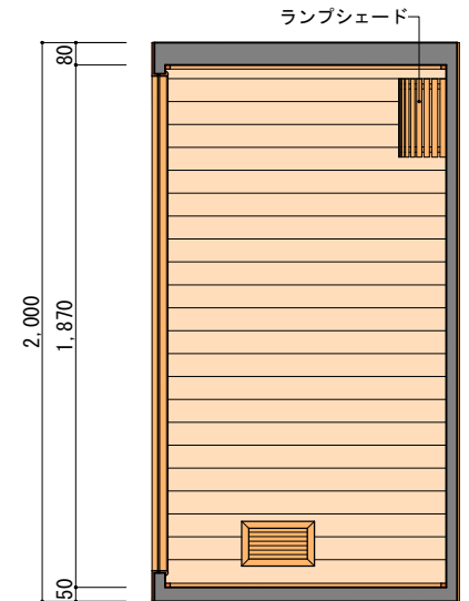
D 展開図 S=1/30
