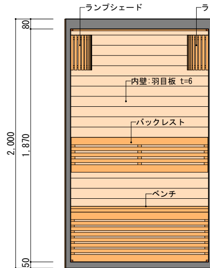
A 展開図 S=1/30
