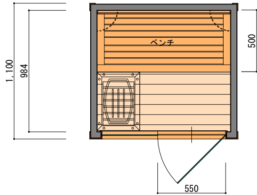
平面図 S=1/30
