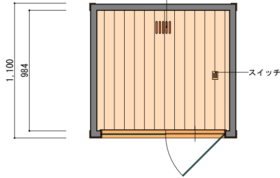
天井伏図 S=1/30
