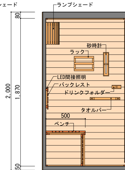
B 展開図 S=1/30
