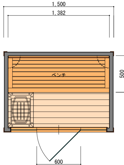
平面図 S=1/30
