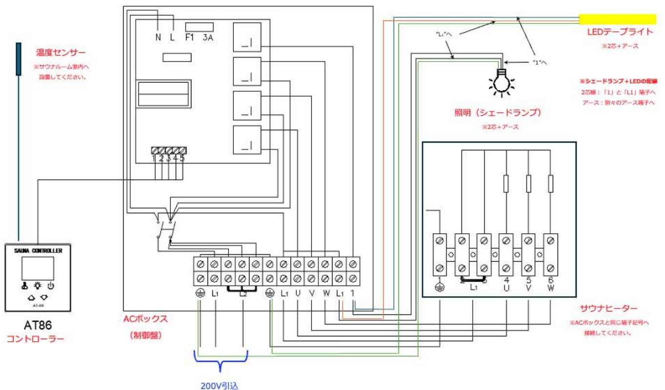
配線図 1
