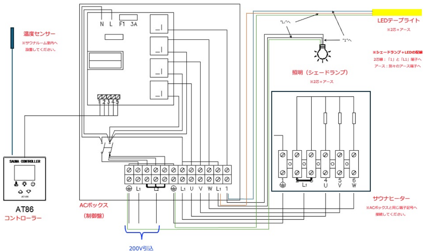
配線図 1
